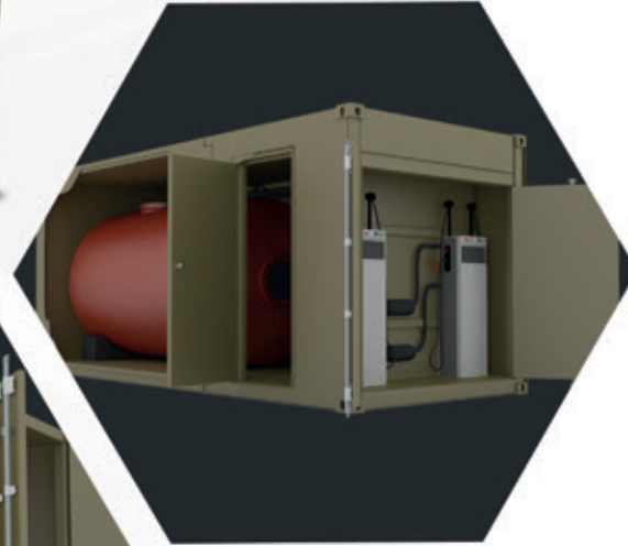
Yakıt Ünitesi Fuel Unit
